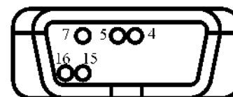
Рис.1. Адресация вилки диагностического кабеля для ВАЗ-ГАЗ-УАЗ (Евро -3/4)
