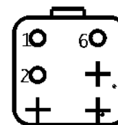
Рис.2. Адресация розетки диагностического кабеля для VDO/STEYR
