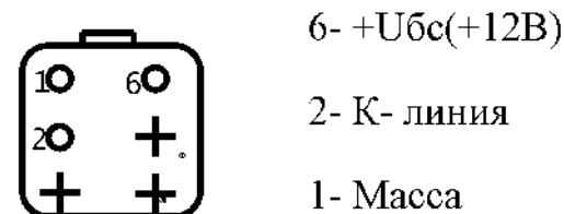
Рис.3. Адресация розетки диагностического кабеля для VDO/ШТАЙЕР
