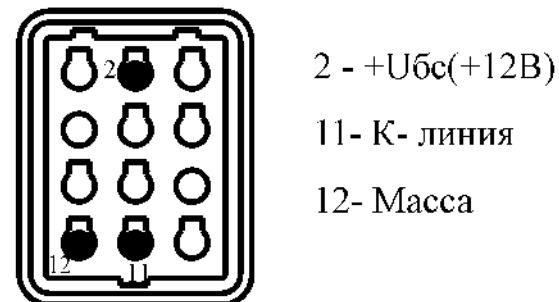
Рис.2. Адресация вилки диагностического кабеля ГАЗ-УАЗ (Евро -0/2 )
