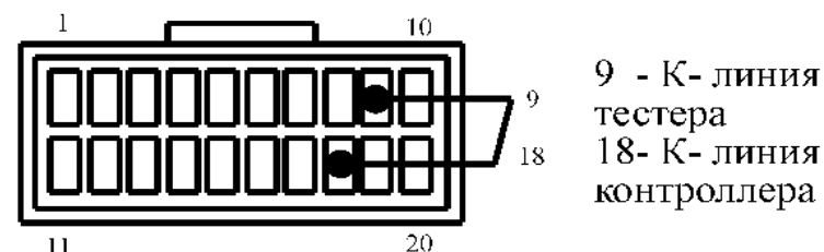
Рис.4. Перемычка на жгутовой розетке соединителя АПС
