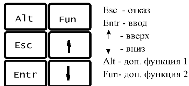
Рис.2. Адресация вилки диагностического кабеля ВАЗ (Евро -0/2 )
