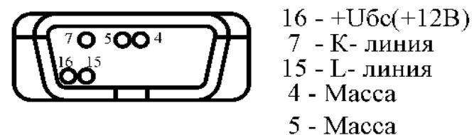
Рис.4. Перемычка на жгутовой розетке соединителя АПС
