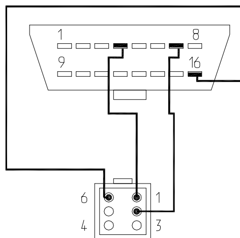
Вид на контакты с лицевой стороны
